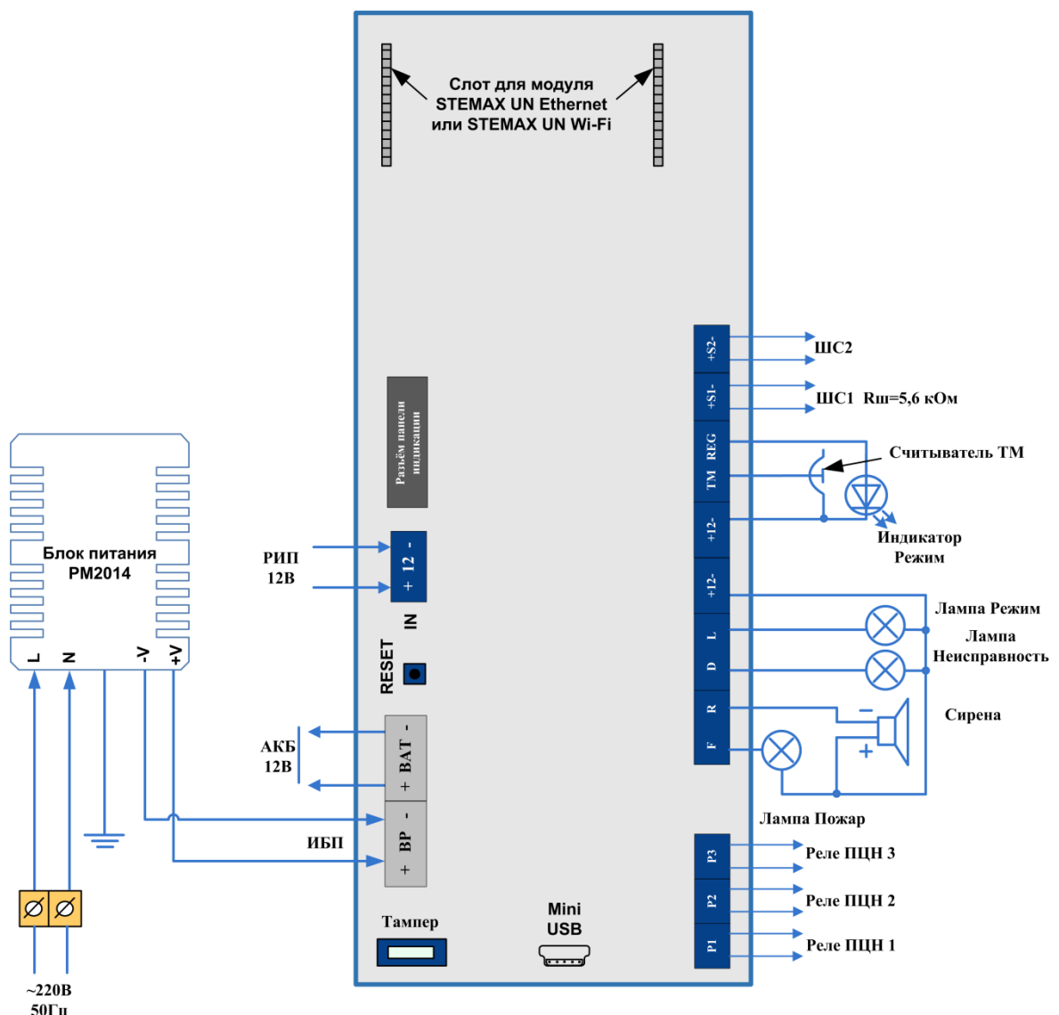
Схема внешних подключений ППКОП STEMAX FX210
