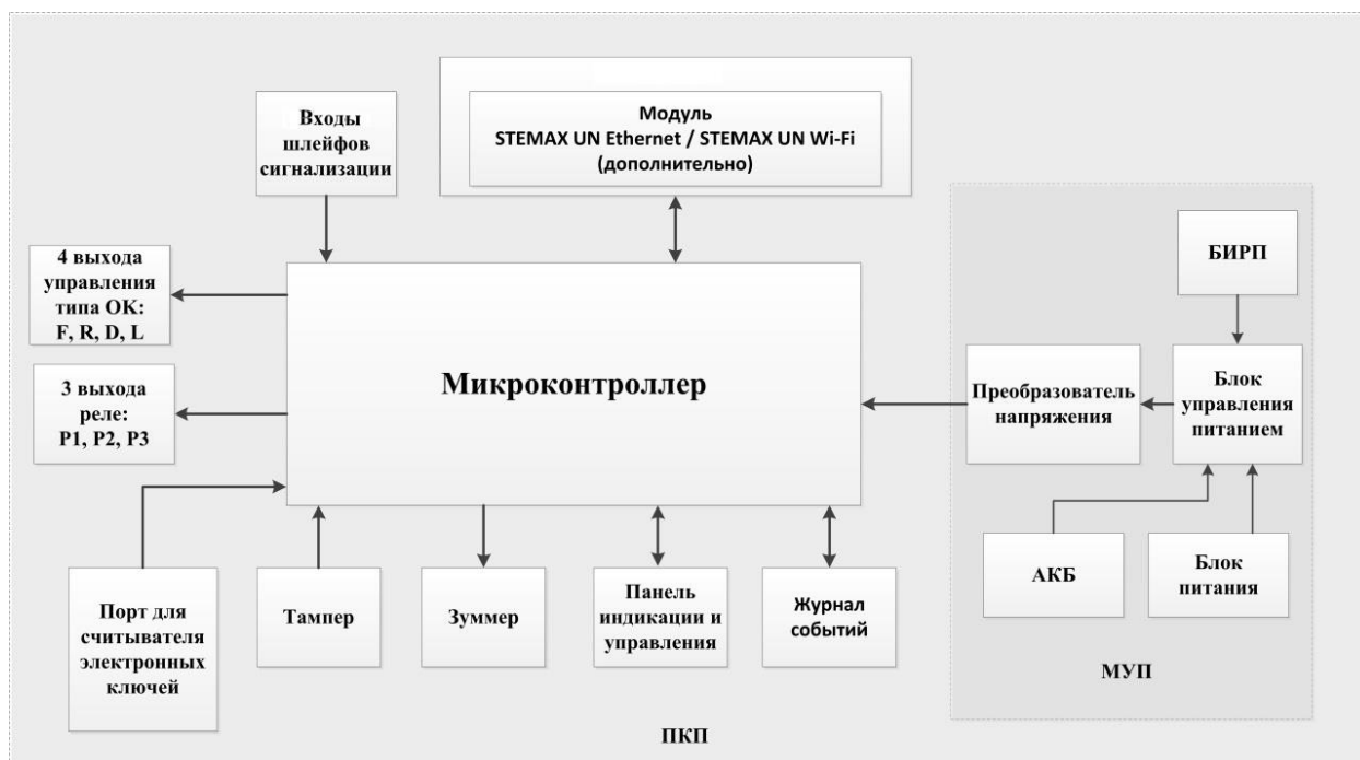
Рис. 3.1. Функциональная схема
