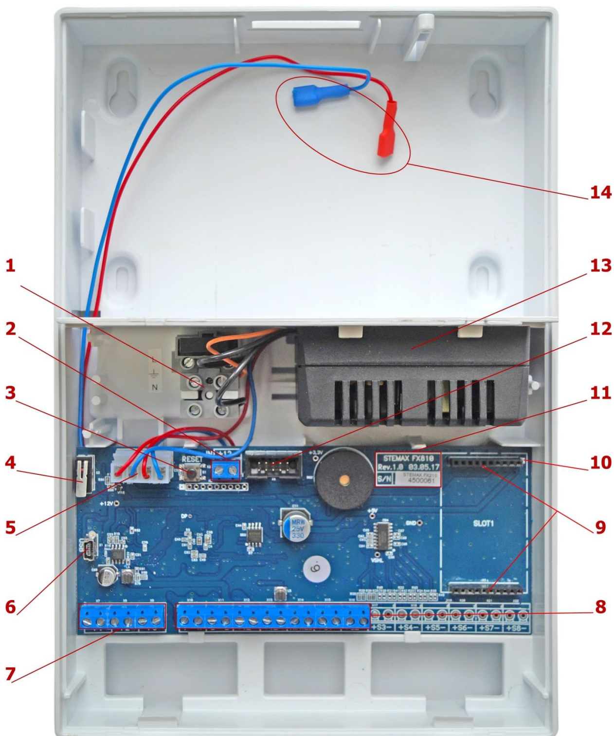
Вид ППКОП STEMAX FX210 со снятой крышкой
