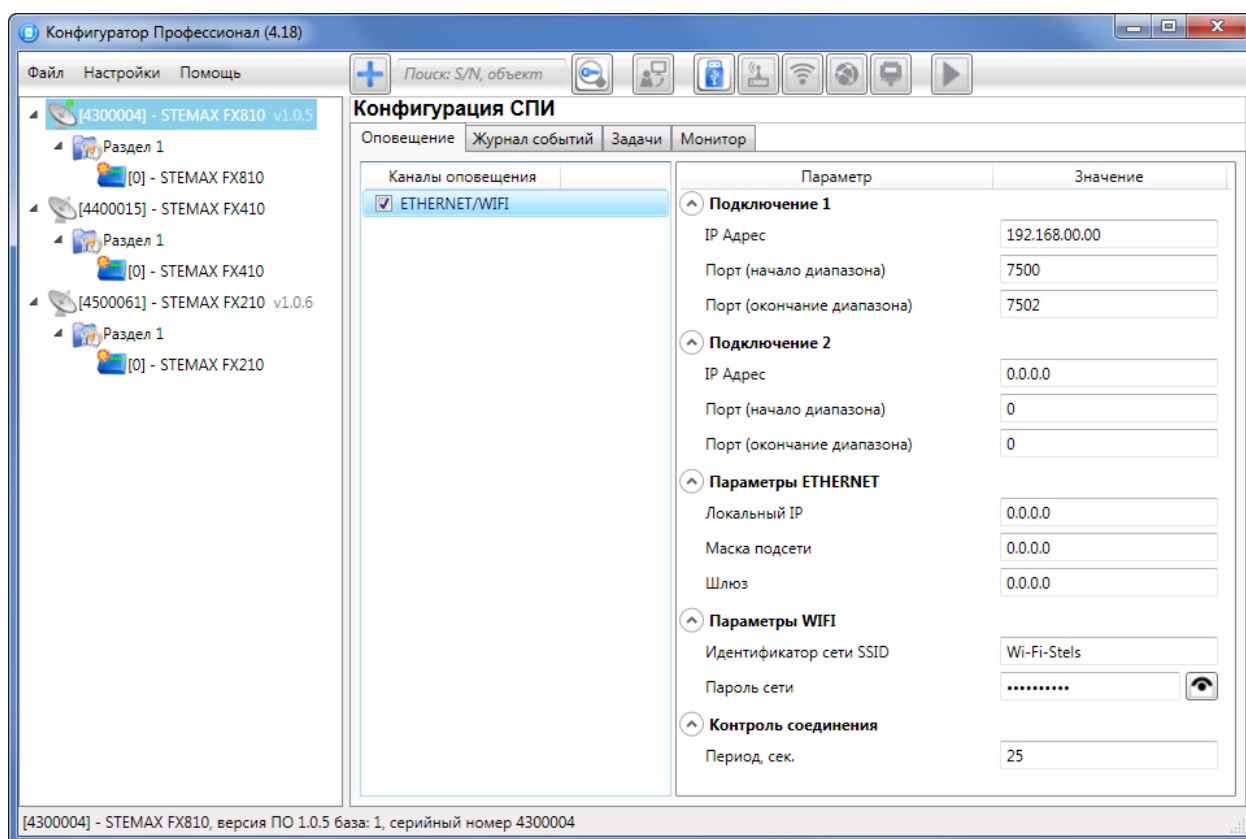
Рис. 8.2. Вкладка Оповещение
