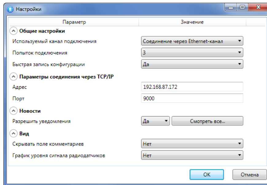
Рис. 6.3. Окно Настройки
