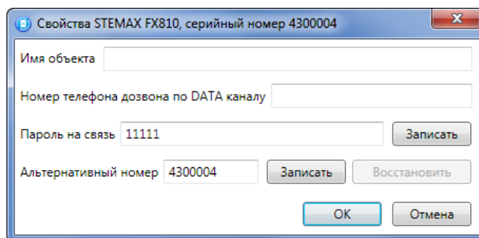
Рис. 12.5. Окно Свойства
