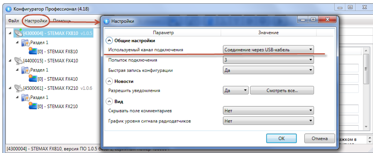
Рис. 6.1. Окно Настройки
