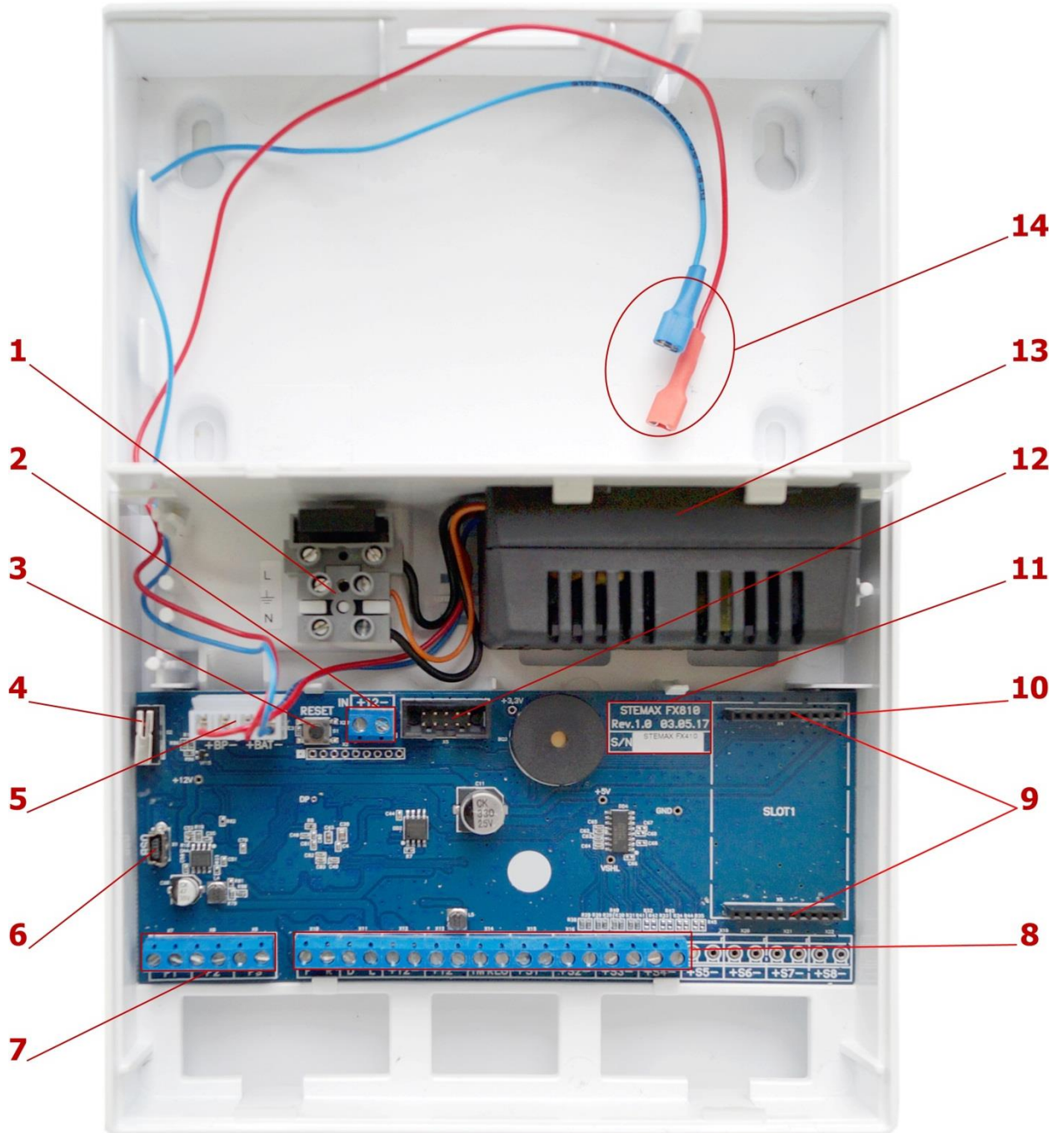
Вид ППКОП STEMAX FX410 со снятой крышкой
