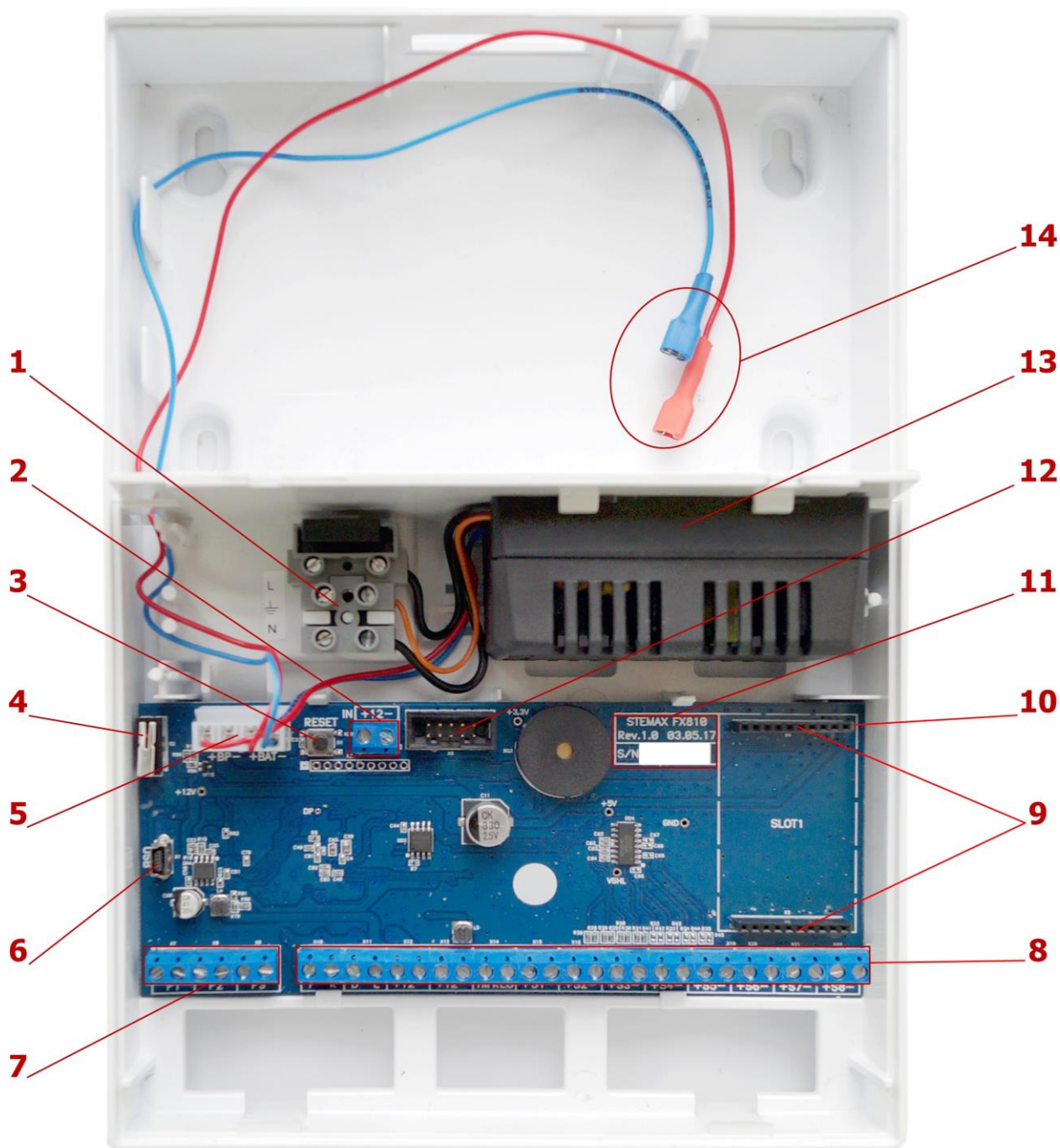
Вид ППКОП STEMAX FX810 со снятой крышкой
