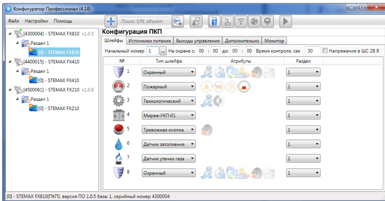
Рис. 10.2. Вкладка Шлейфы
