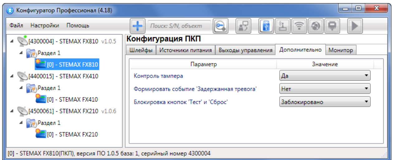
Рис. 10.7. Вкладка Дополнительно
