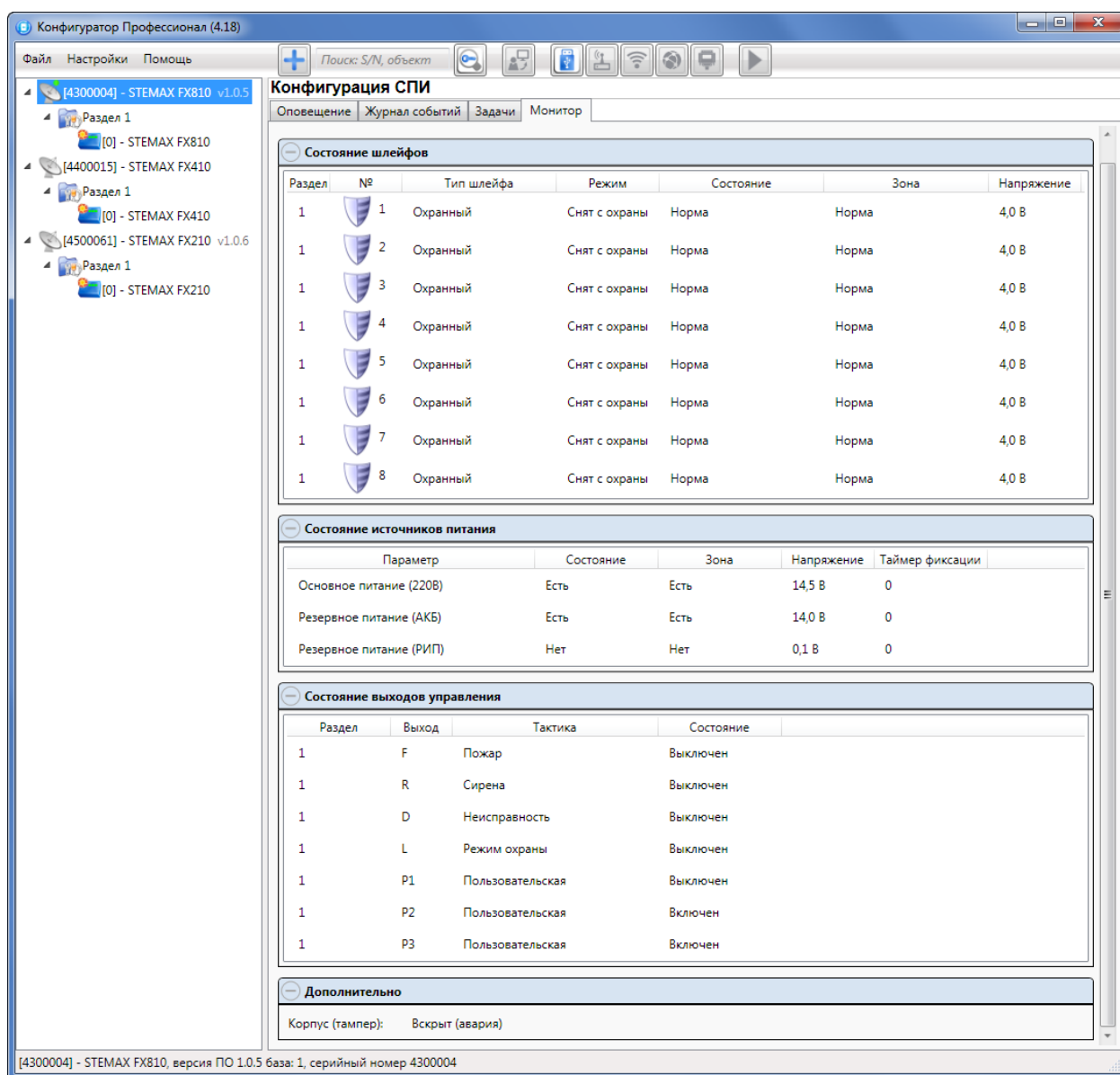
Рис. 8.6. Вкладка Монитор
