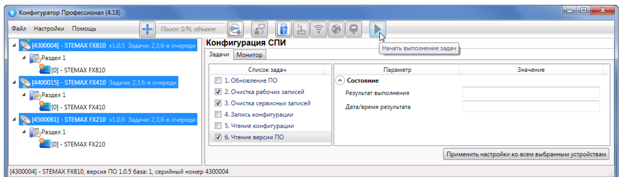
Рис. 8.5. Вкладка Задачи
