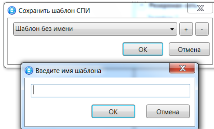
Рис. 12.3. Сохранение шаблона
