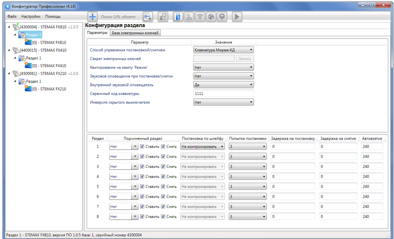
Рис. 9.2. Вкладка Параметры
