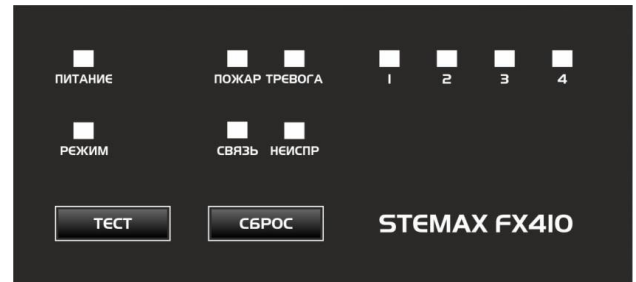
Рис. 3.7. Панель индикации ППКОП STEMAX FX410
