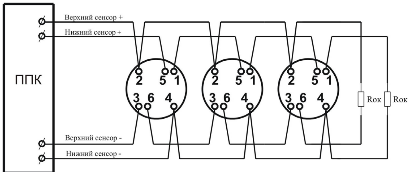
Схема подключения извещателей ИП-2.4 к ППК с постоянноточковым питанием шлейфов в режиме I_{тр} > 9\text{мА}
