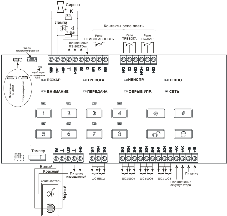
Рисунок 8 – Монтажная схема прибора
