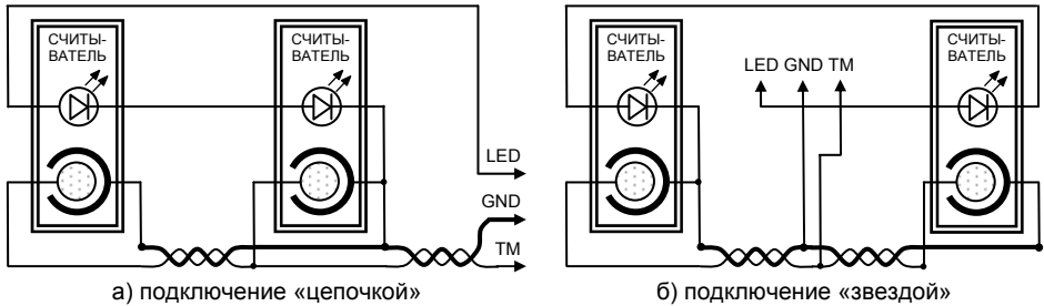
Рисунок 7 – Подключение двух считывателей
