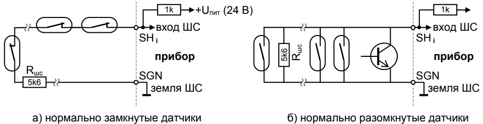
Рисунок 5 – Примеры монтажа охранных шлейфов
