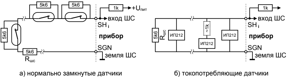
Рисунок 6 – Примеры монтажа пожарных шлейфов
